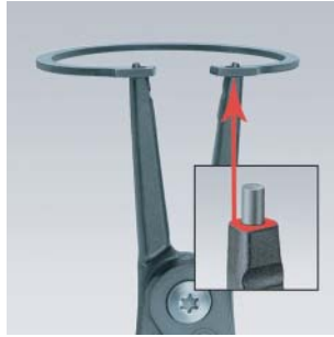
Suuret kontaktipinnat estävät lukkorengaan tahattoman irtoamisen
